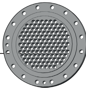
WÄRMETAUSCHERPLATTE
